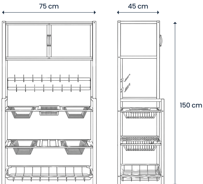
TAMPAK DEPAN
